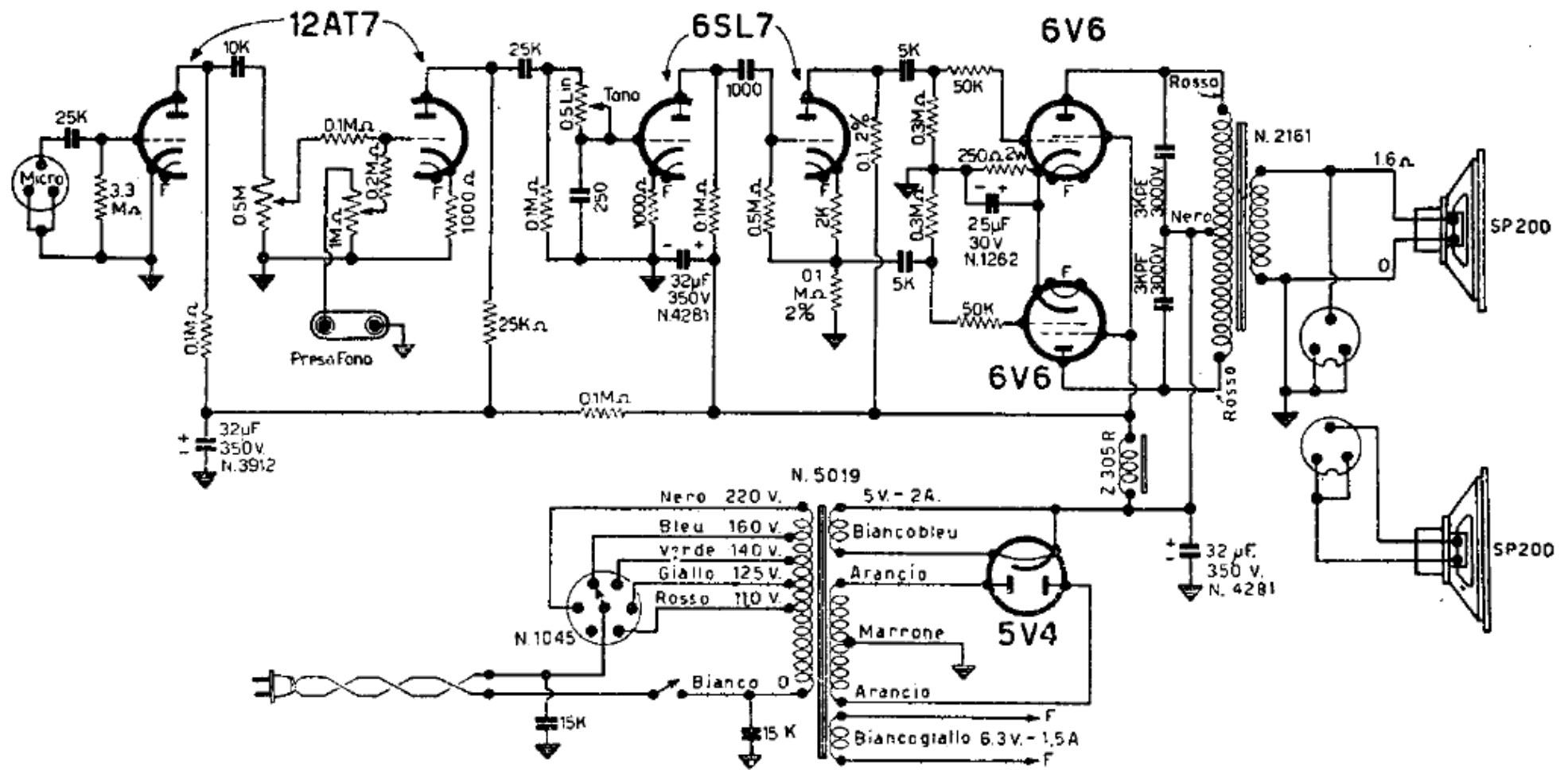
AMPLIFICATORE G. 206-V
